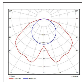
Lichtdiagram SRTI
