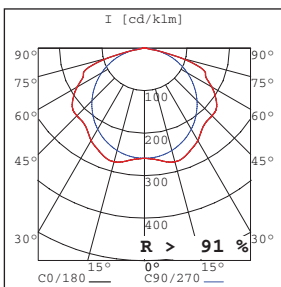
Lichtdiagram RT1/2
