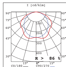
Lichtdiagram RTL153
