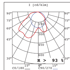
Lichtdiagram S1/2-AB
