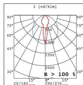
Lichtdiagram S1-DH
