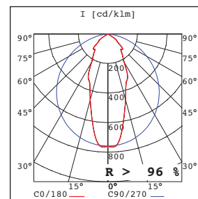
Lichtdiagram S2-DH
