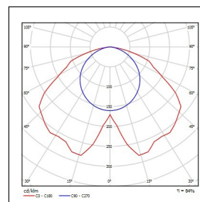
Lichtdiagram SRT1/2-B
