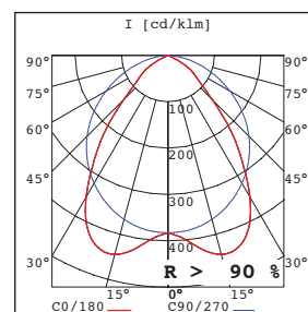
Lichtdiagram S1/2-BH
