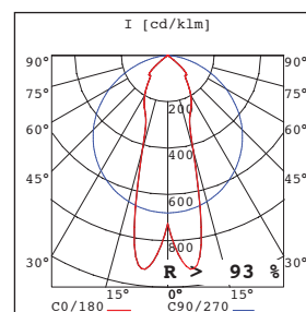
Lichtdiagram S1-DH
