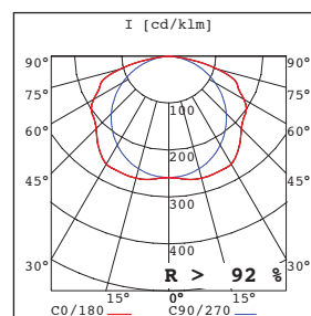
Lichtdiagram RTW1/2-B
