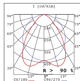
Lichtdiagram SW1/2-B
