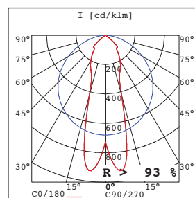
Lichtdiagram SW1-DH
